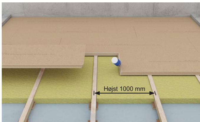
Figur 4 Spaandex K-gulvplader lagt med flyvestød og i forbandt med en forskydning på mindst 450 mm. Strøafstand højst 1000 mm, se tabel 1.
